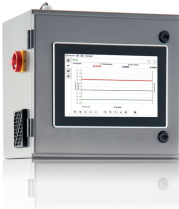
Online-Messwertverlauf über 12 Stunden von Erdgas am Standort Union Instruments GmbH, Karlsruhe
